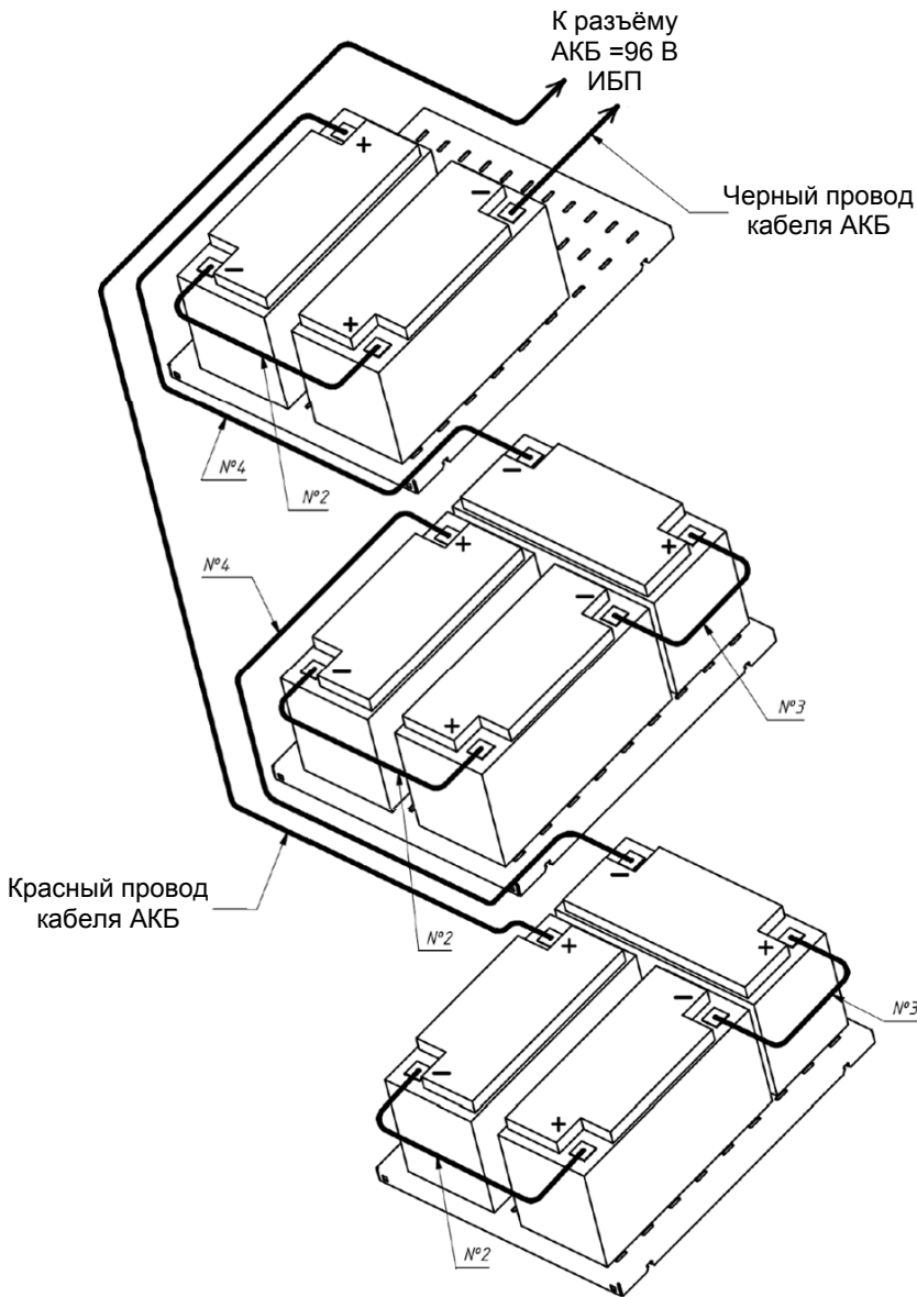
Рисунок 1. Размещение АКБ на полках шкафа и соединение их перемычками.
