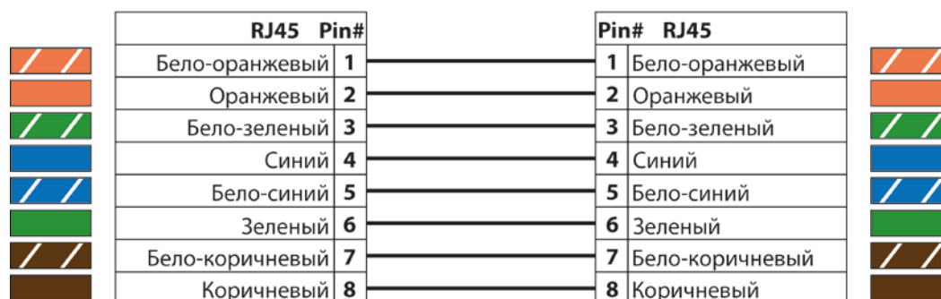
Рисунок 17. Прямая схема обжима кабеля
