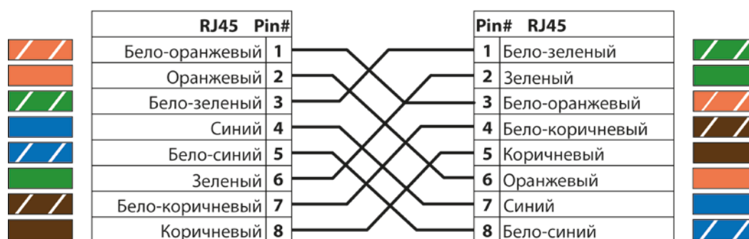
Рисунок 16. Кроссовая схема обжима кабеля
