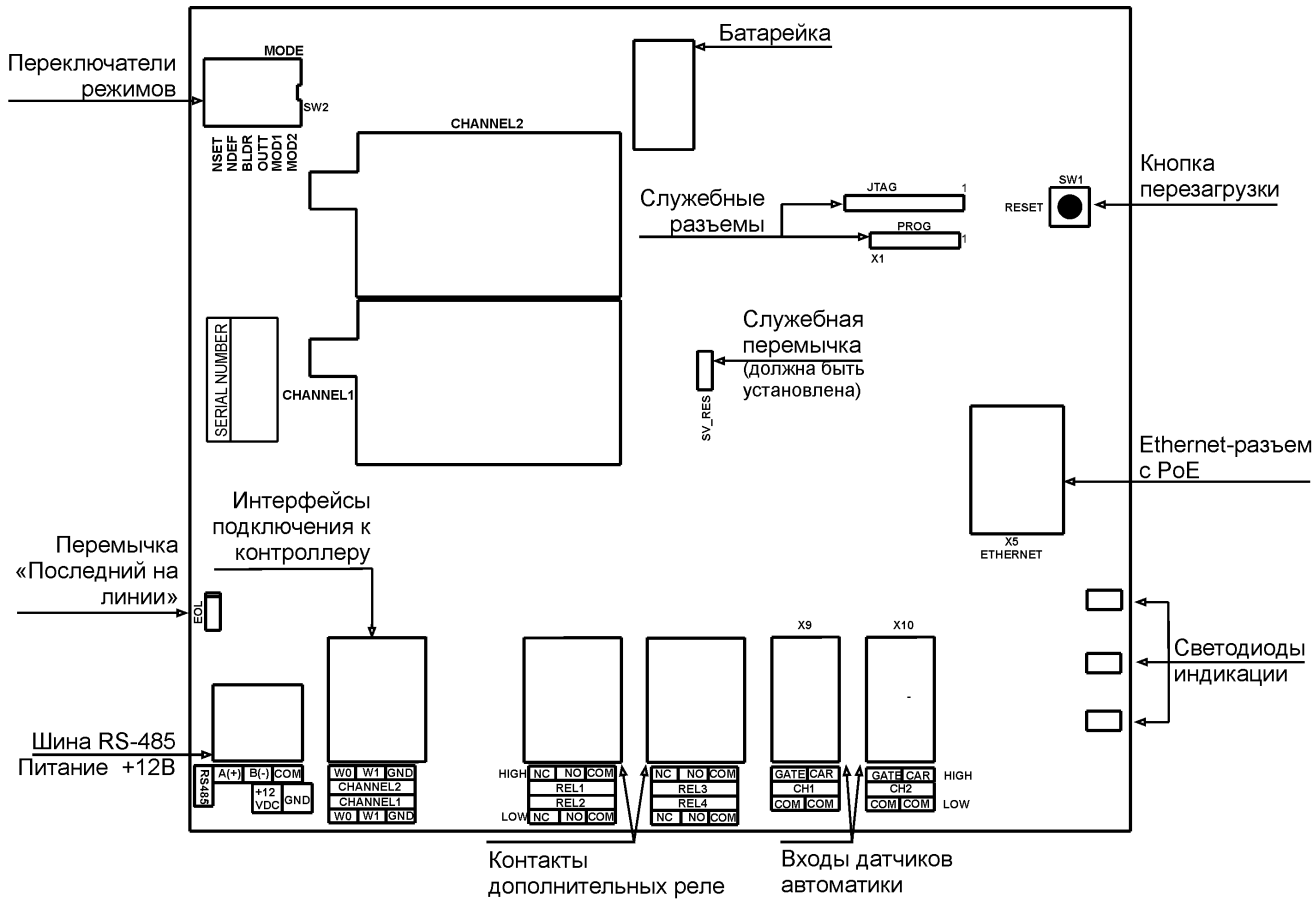
Рисунок 2. Схема основных элементов считывателя PR-G07.N
