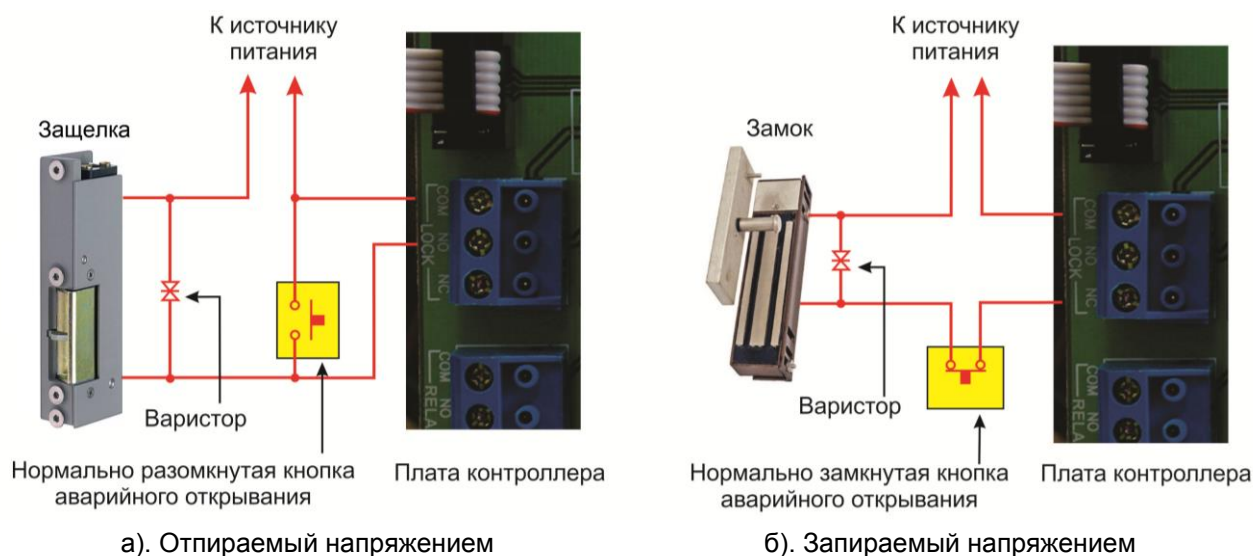
Рисунок 11. Подключение замка двери к контроллеру
