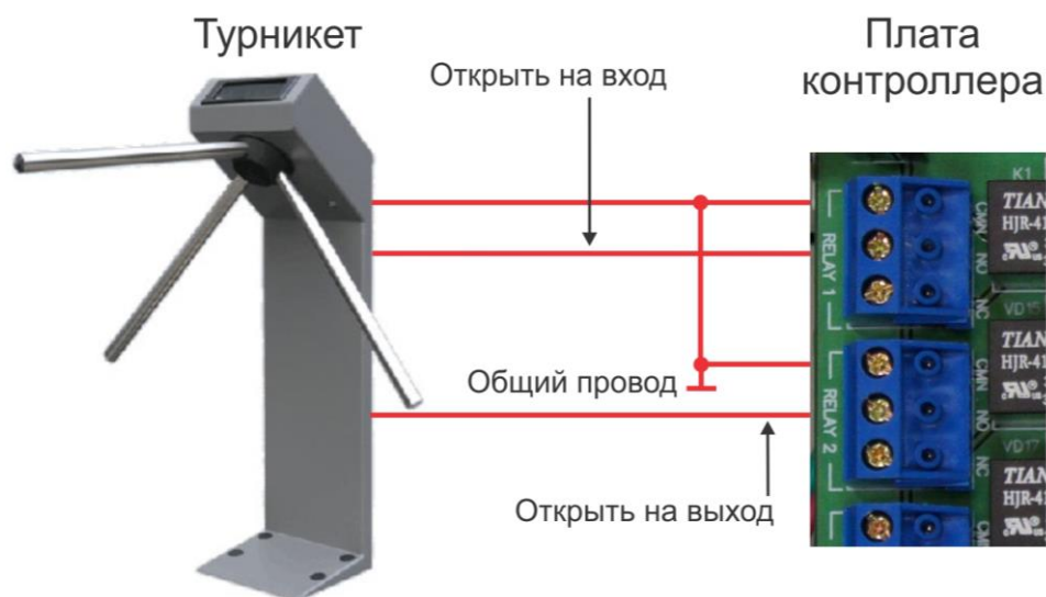
Рисунок 13. Управление турникетом
