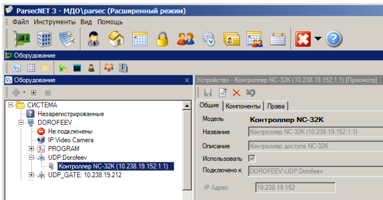
Рисунок 31. Настройка контроллера в ParsecNET 3
