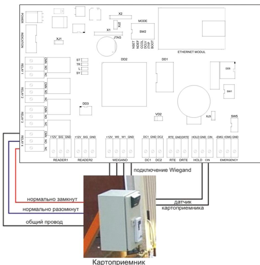
Рисунок 16. Подключение картоприемника
