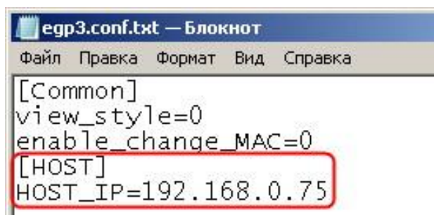
Рисунок 29. Принудительное назначение сетевого адреса
