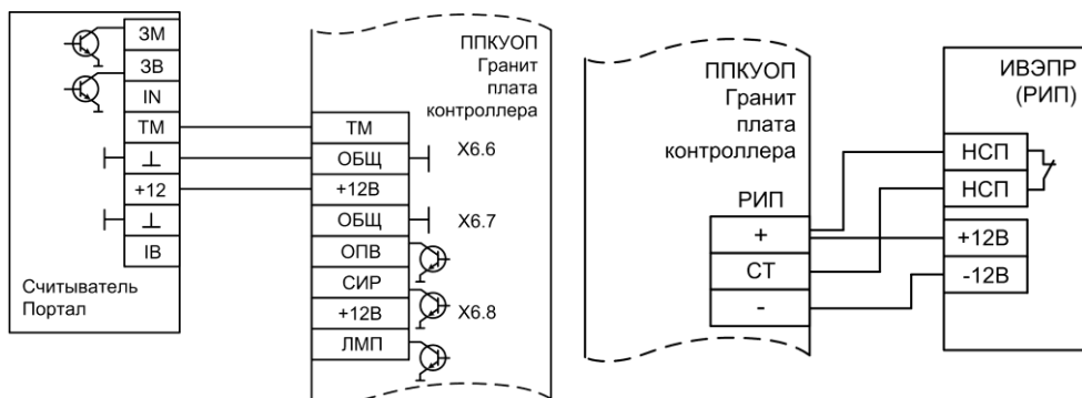
Рис.Б5 Схема подключения источника внешнего электропитания резервированного (РИП)
