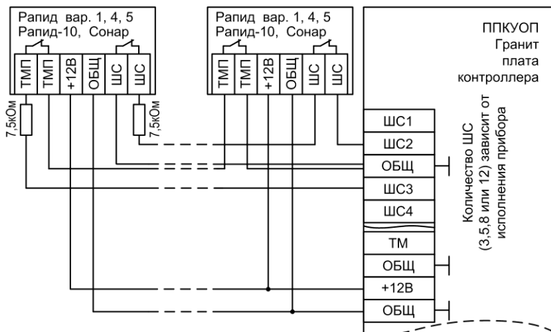
Рис.Б3 Схема подключения охранных извещателей Рapid вар.1,4,5, Рapid-10, Сонар (тампер подключён к отдельному ШС)
