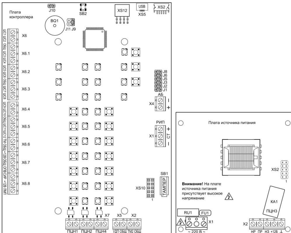
Рис.1 Внешний вид платы контроллера Гранит-12 и платы источника питания
