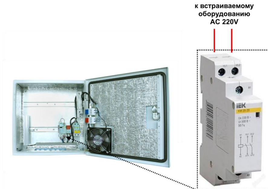
Рис. 22 Точка подключения встраиваемого оборудования к сети 220V переменного тока внутри уличной станции с «теплым» пуском на примере модели OS-44H2
