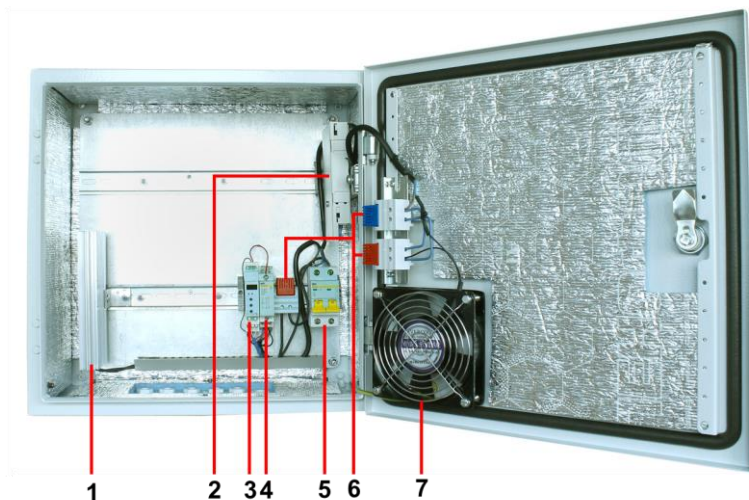
Рис. 10 Уличная станция OS-44H2, внутренние элементы
