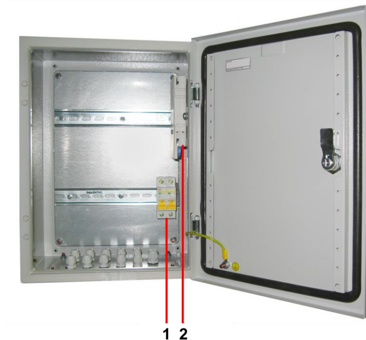
Рис.16 Уличная станция OS-341, внутренние элементы
