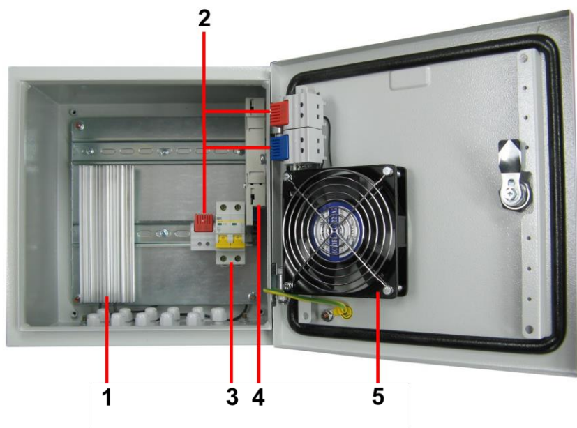
Рис.14 Уличная станция OS-33T1 с термостабилизацией, внутренние элементы
