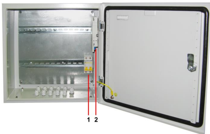
Рис.4 Уличная станция OS-441, внутренние элементы
